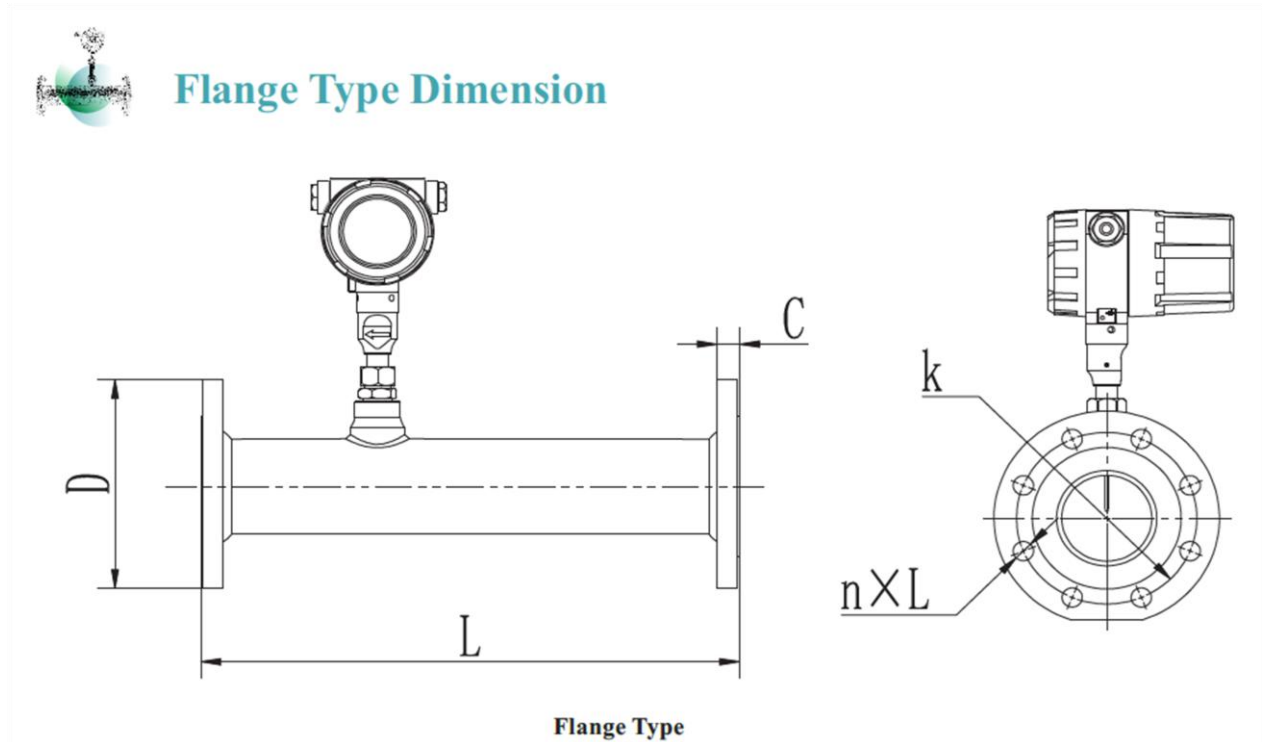
DIN PN16 Flange (Unit: mm)
